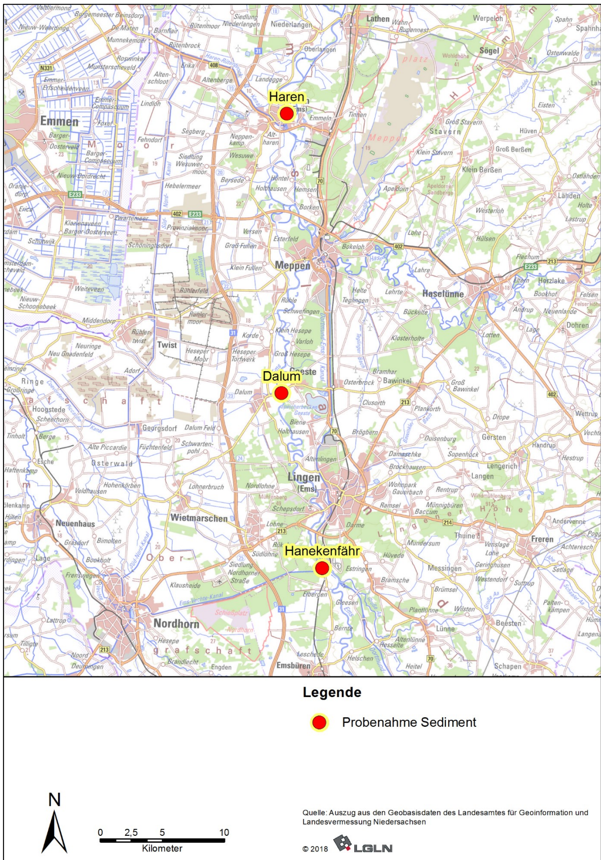
Abb. 2-7: Probenahmeorte für Sedimentproben (Hanekenfähr (Ems km 84,7), Dalum (Ems km 106,3), Haren (Ems km 179))
