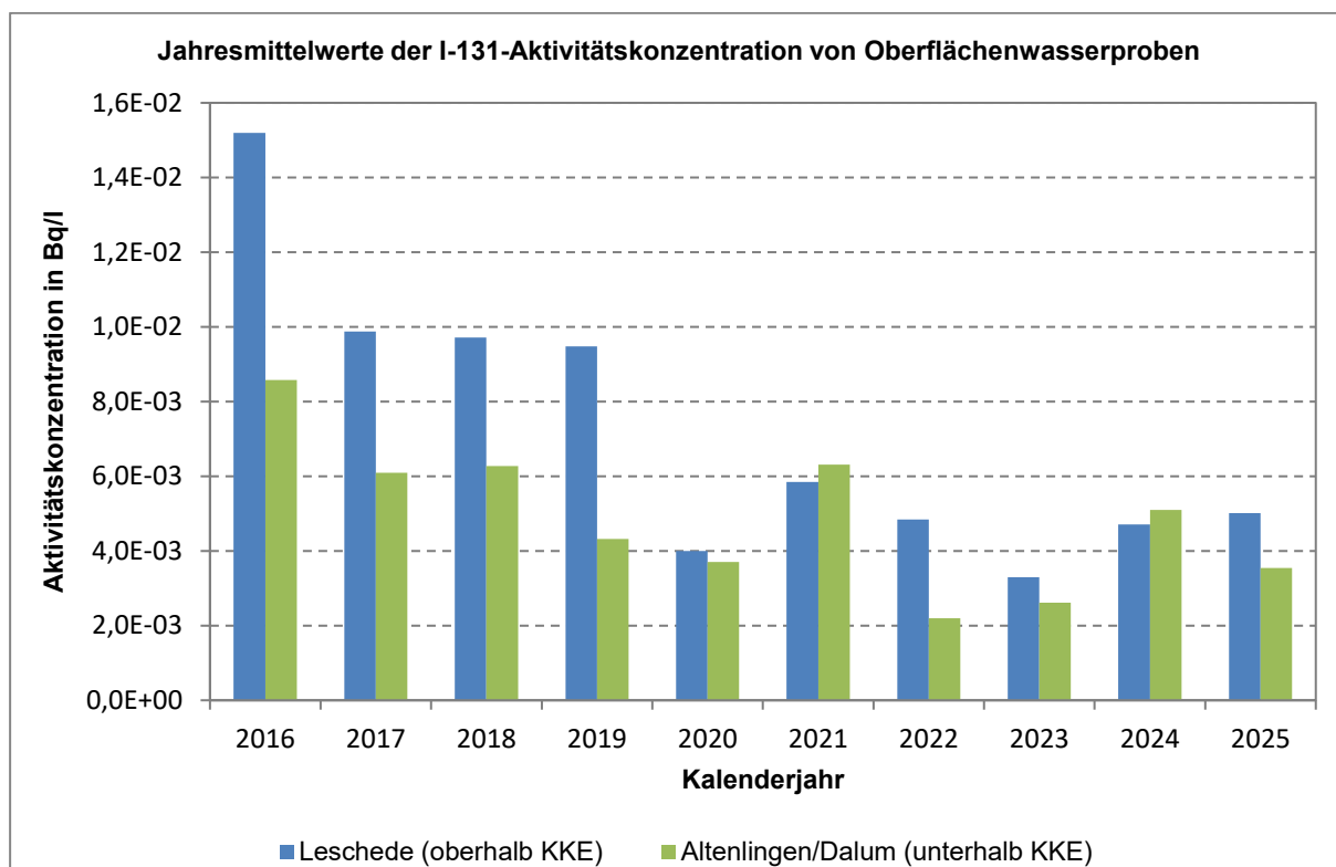
Abb. 4-11: I-131-Aktivitätskonzentration im Jahresmittel von Oberflächenwasserproben oberhalb und unterhalb der Anlage in der Ems
