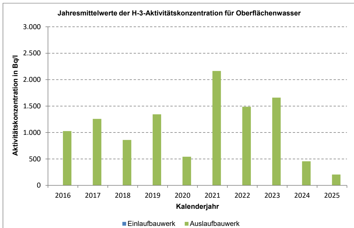
Abb. 4-7: H-3-Aktivitätskonzentration im Jahresmittel von Oberflächenwasserproben im Einlauf- und Auslaufbauwerk der Anlage
