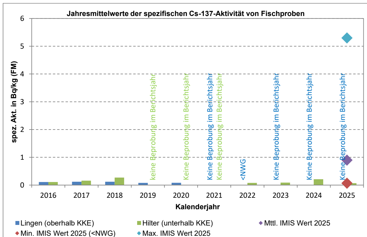
Abb. 4-14: Spezifische Cs-137-Aktivität im Jahresmittel von Fischproben
