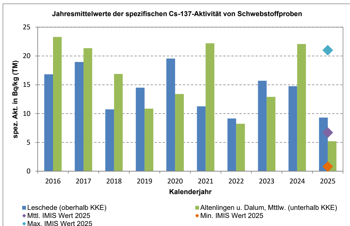
Abb. 4-13: Spezifische Cs-137-Aktivität im Jahresmittel von Schwebstoffproben
