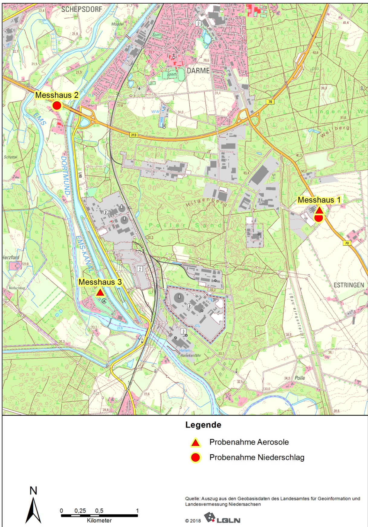
Abb. 2-3: Probenahmeorte für Aerosol- und Niederschlagsproben (Messhaus 1 bis 3)
