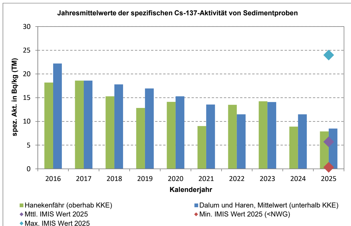
Abb. 4-12: Spezifische Cs-137-Aktivität im Jahresmittel von Sedimentproben
