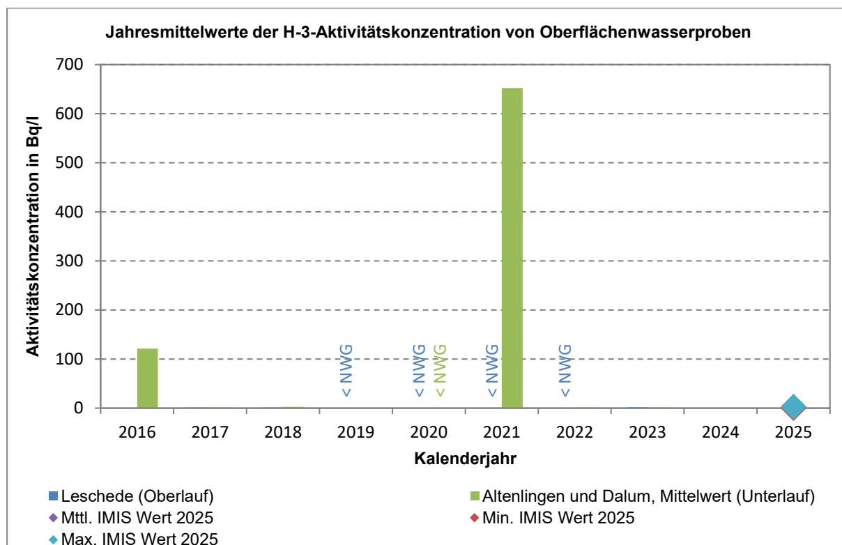
Abb. 4-8: H-3-Aktivitätskonzentration im Jahresmittel von Oberflächenwasserproben oberhalb und unterhalb der Anlage in der Ems
