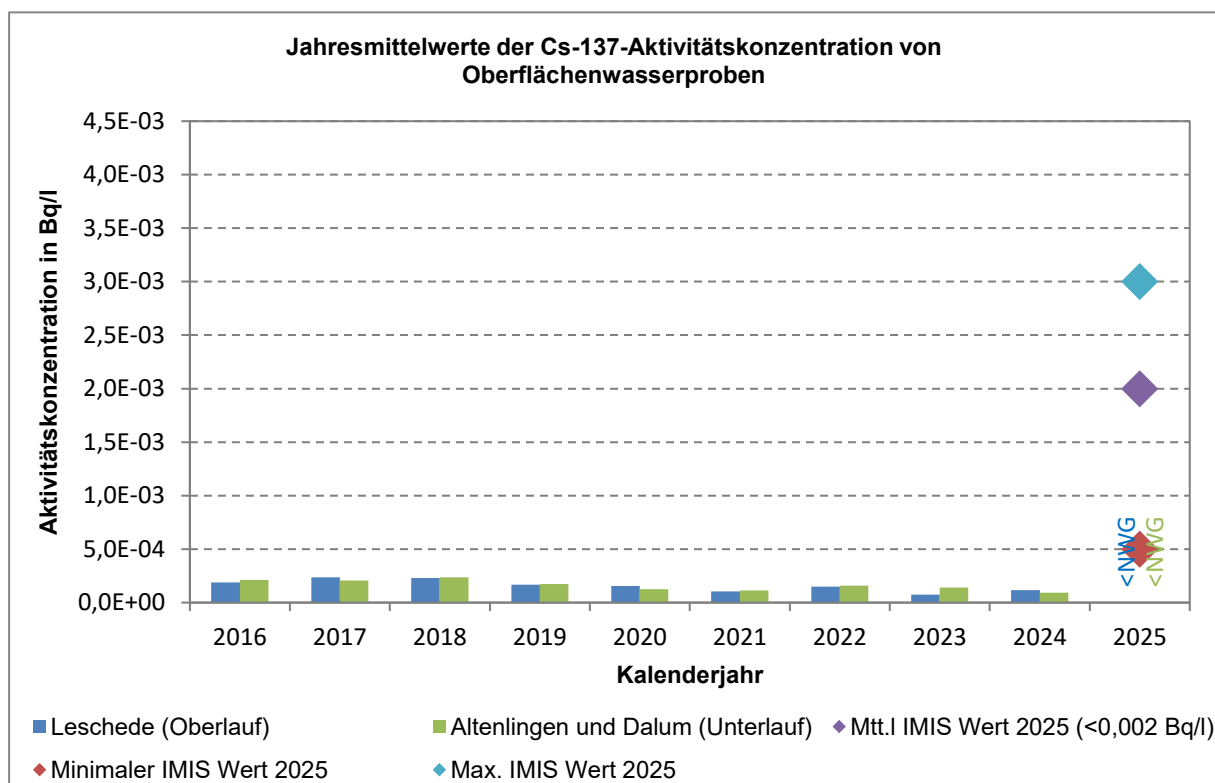
Abb. 4-10: Cs-137-Aktivitätskonzentration im Jahresmittel von Oberflächenwasserproben oberhalb und unterhalb der Anlage in der Ems
