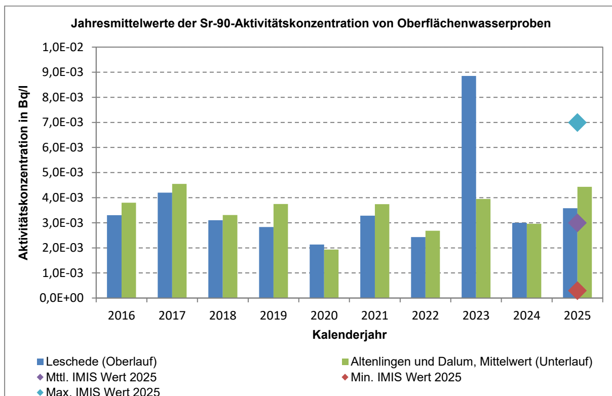
Abb. 4-9: Sr-90-Aktivitätskonzentration im Jahresmittel von Oberflächenwasserproben oberhalb und unterhalb der Anlage in der Ems
