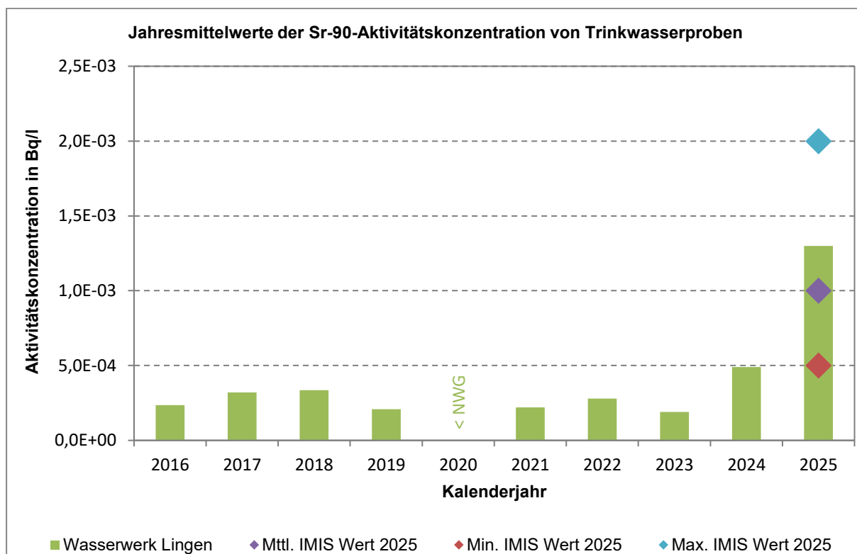
Abb. 4-16: Sr-90-Aktivitätskonzentration im Jahresmittel von Trinkwasserproben
