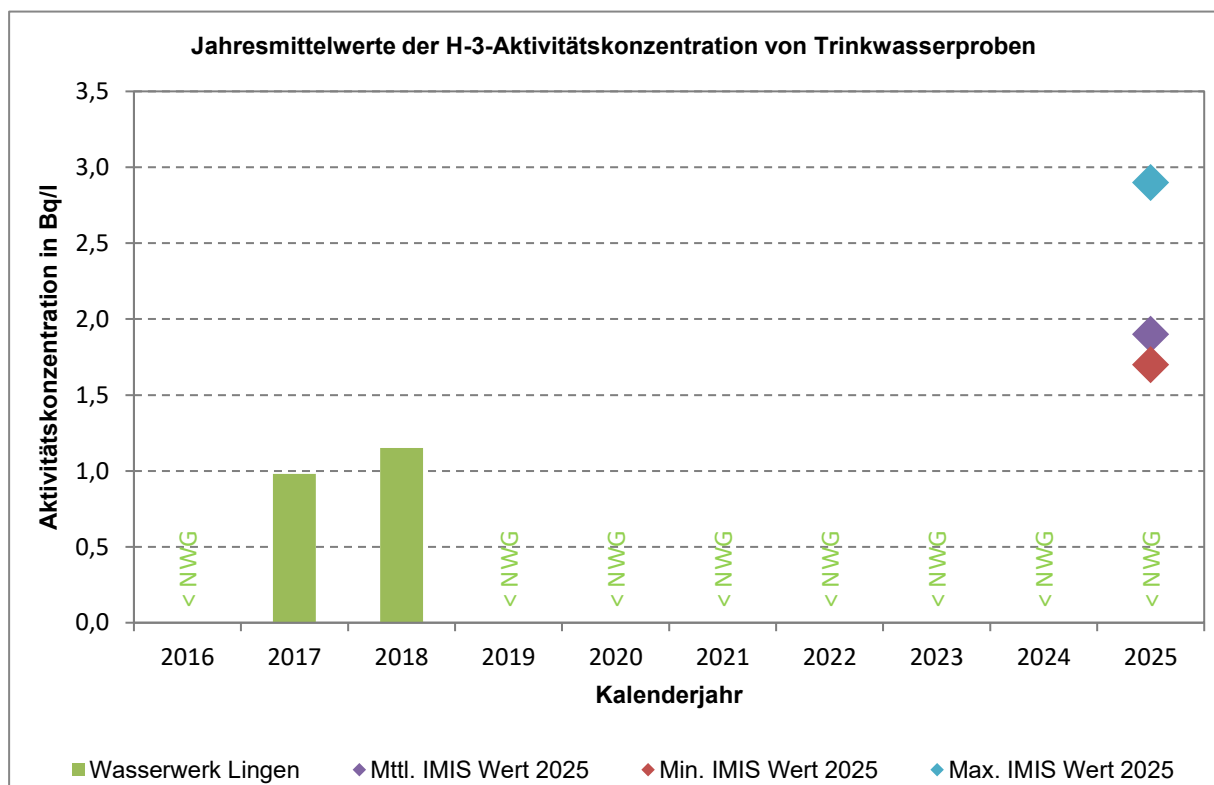
Abb. 4-15: H-3-Aktivitätskonzentration im Jahresmittel von Trinkwasserproben
